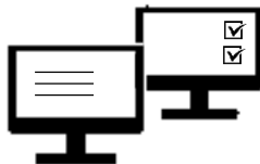
管理画面
